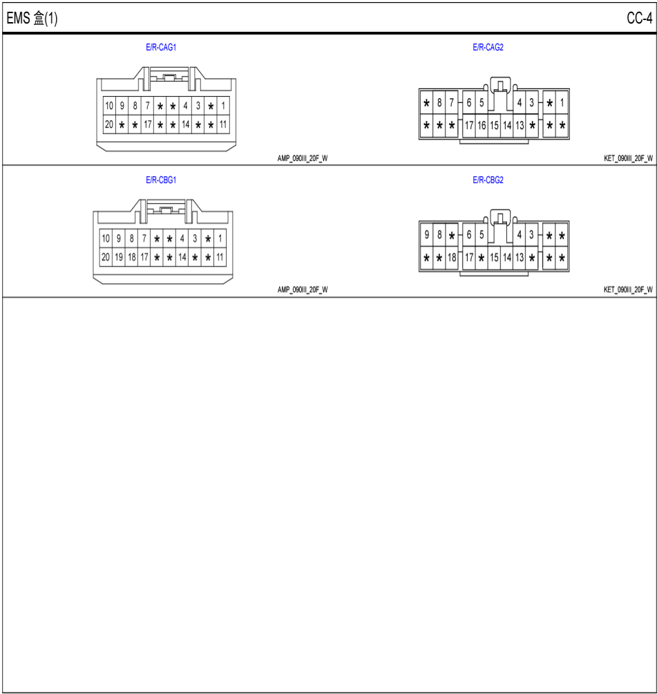
室内接线盒 & 短接连接器
